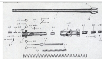
MG 34, Einzelteil: Lauf mit Verschluss
