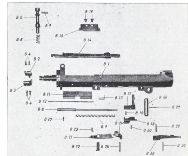
MG 34, Einzelteile: Gehäuse
