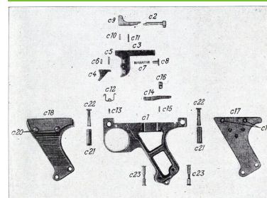
MG 34, Einzelteile: Griffstück
